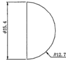
图 1 A型冲头
