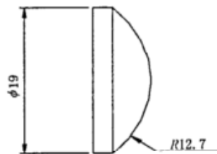
图 2 B型冲头
